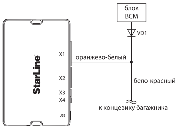
Схема 3. Подключение концевого багажника
