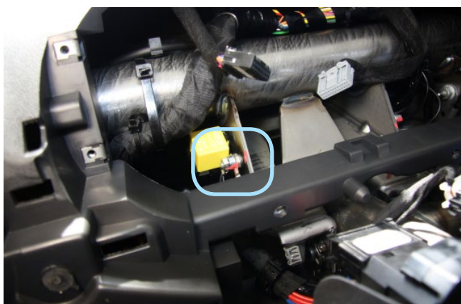
Фото 3.1. Подключение массы
