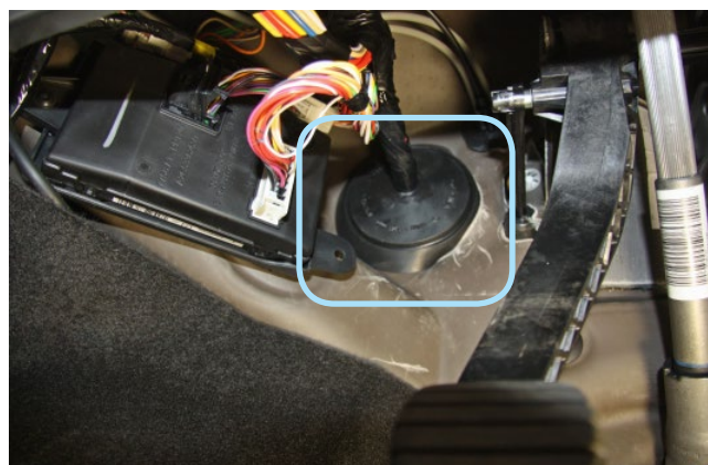
Фото 2.4. Штатный уплотнитель. Вид со стороны салона
