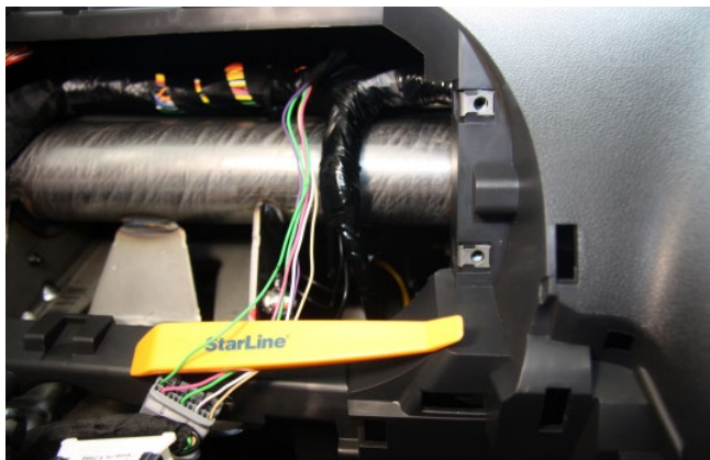
Фото 3.3. Контроль концевиков дверей (зелёный)
